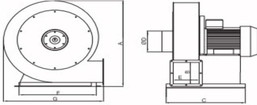
Şekil 2.28: Taşıyıcı fan kısımları
