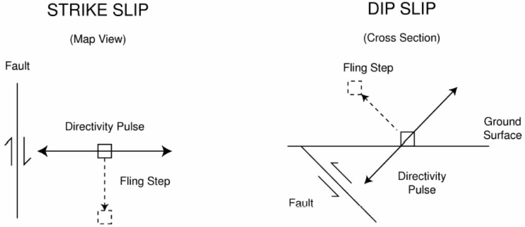
řekil 3.10: Kayma eęimi ve kayma yönü faylanması için, yer deęiřim ( Fling step), Pals yönleri( Directivity)
