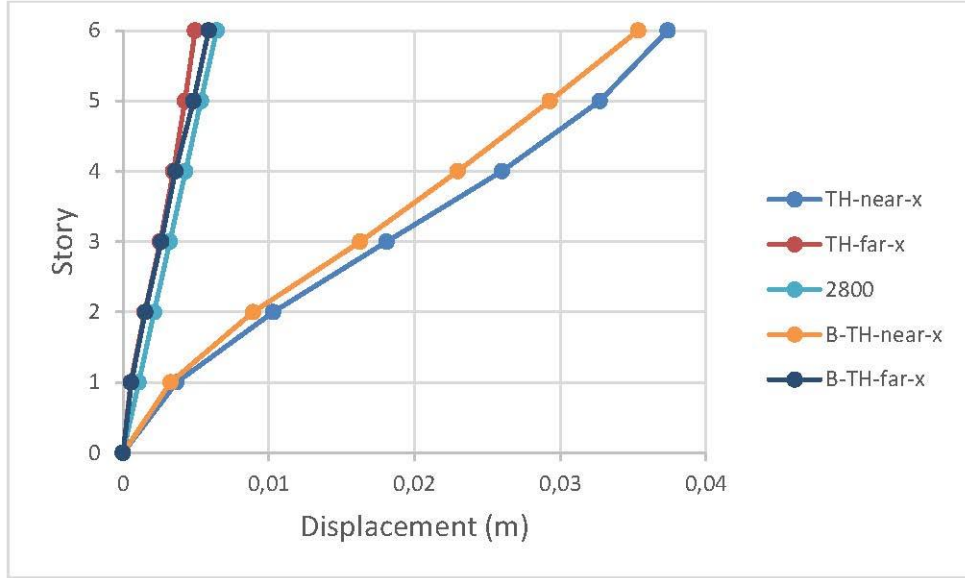
Şekil 4.3: 6 katlı yapıların X yönünde yer değişim karşılaştırması
