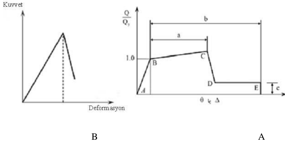
Şekil 2.3: A) Elastik elementler davranış eğimi B) kırılğan elementler davranış eğimi(7)
