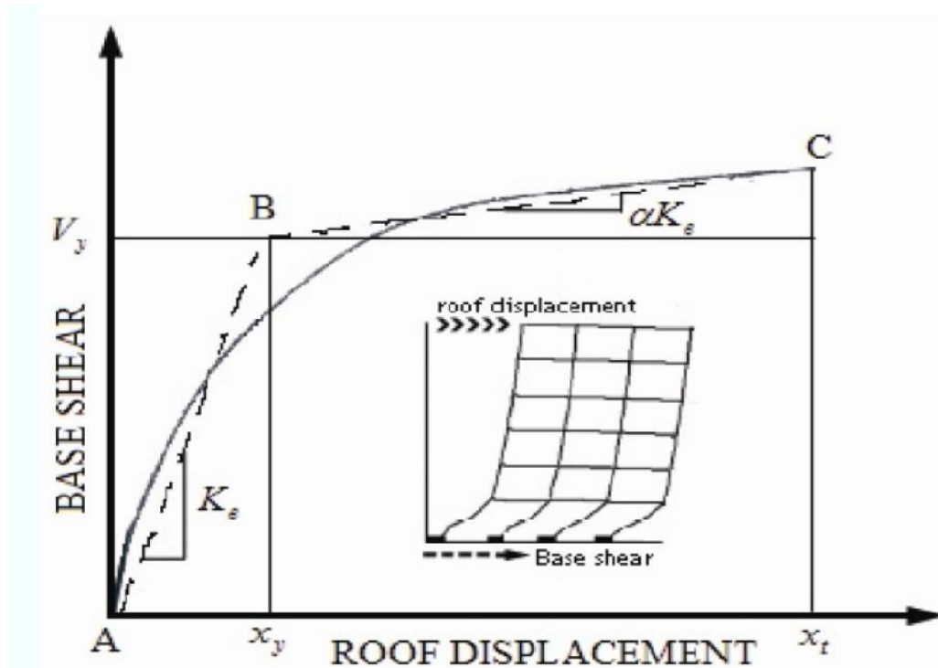
Şekil 3.6: Kuvvet Yer Değişim Diyagramı
