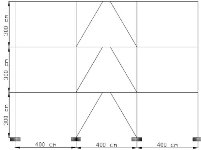
Şekil 2.2: 3 ağızlı ve 2 çerçevesi geometri
