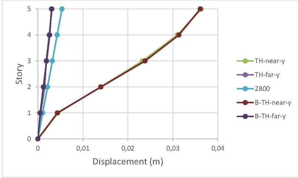
Şekil 4.2: 5 katlı yapıların Y yönünde yer değişme karşılaştırması
