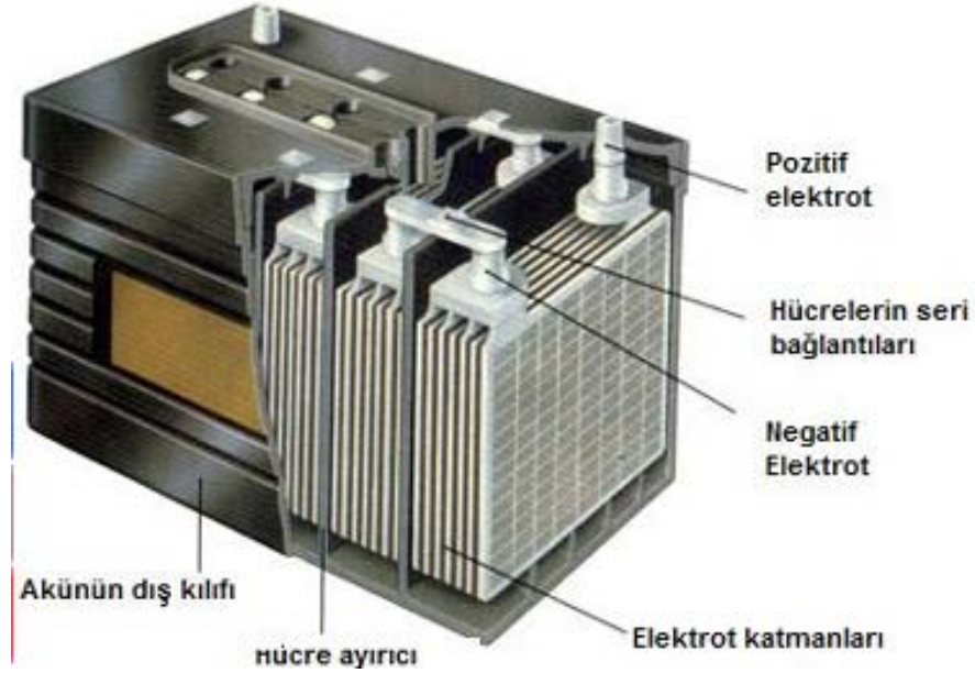
Şekil 6.9: Akümülatör
