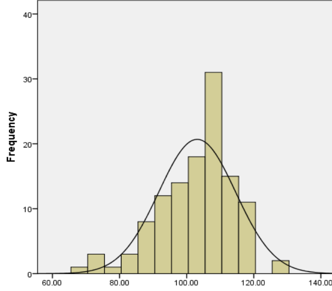
Şekil 4.6: Normallik Değerlendirmesi
